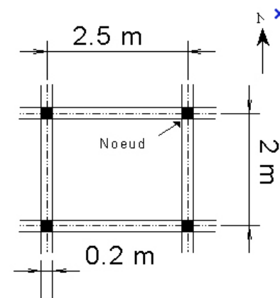
Réseau Hartmann
